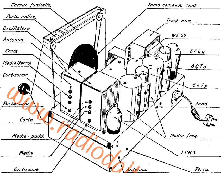
COMPAGNIA GENERALE DI ELETTRICITÀ. - Mod. 1331 e 1332. Posizione delle parti, valvole, compensatori e nuclei ferromagnetici.
