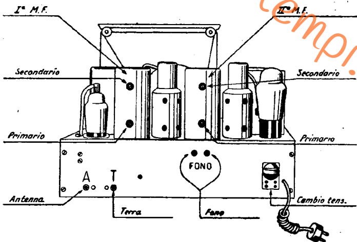
COMPAGNIA GENERALE DI ELETTRICITÀ. - Mod. 1331 e 1332. Posizione compensatori medie frequenze.
