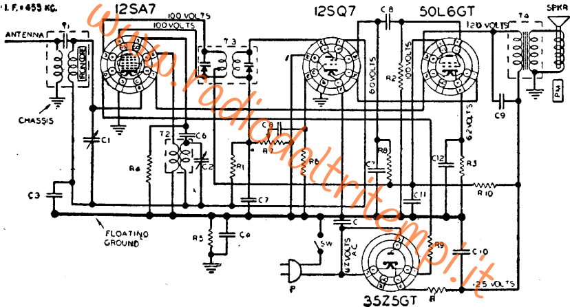
Fig. 6.1. - Esempio di minuscola supereterodina americana.
